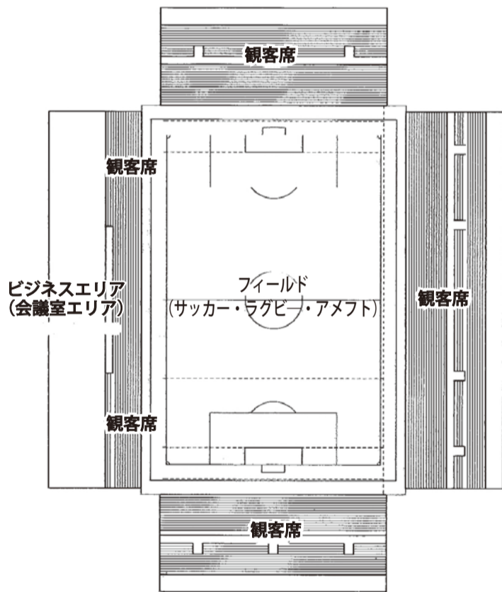
【3階平面図】
